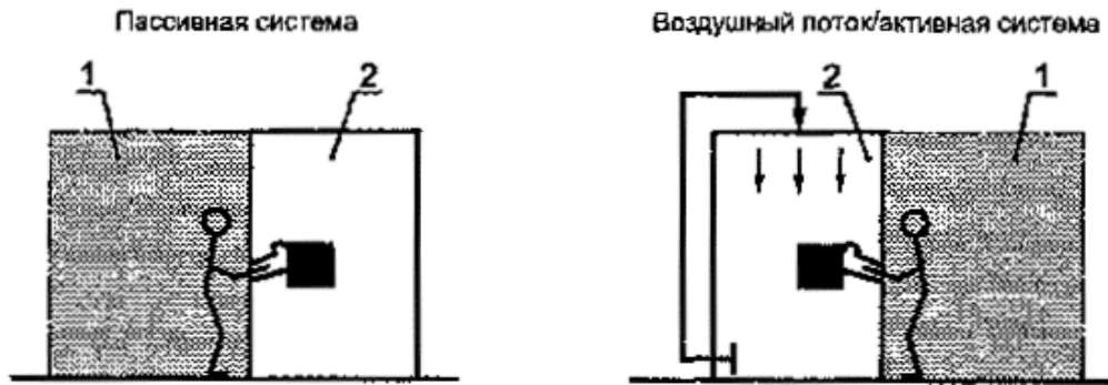
Рисунок А.5 - Принципы организации чистых зон с использованием физического барьера защиты продукта и персонала
